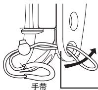
安装示意图
