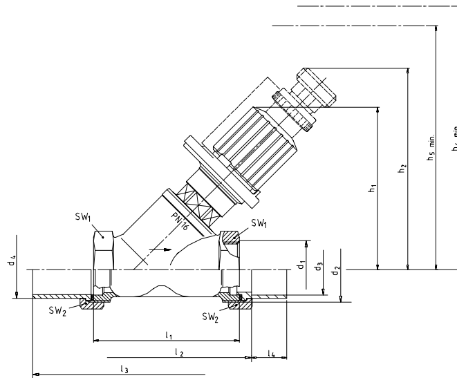
Fig. 3. Kombi-3-plus BLUE
