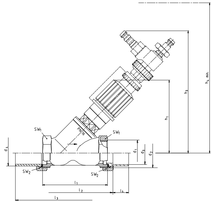
Fig. 2. Kombi-3-plus RED
