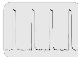
②④ A-Bboard A26 Pin 10 - 5.04V p-p NTSC-HD2
