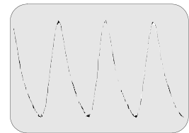
③⑩ A-Bboard A26 Pin 19 - 2.44V p-p FSC
