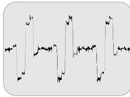
33 A-Board A26 Pin 28 - 0.91V p-p Pr
