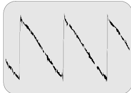
⑫ A-Board A6 Pin 16 - 1.86V p-p V.L. (NECH PRO)
