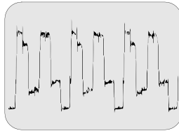
38 A-Board A26 Pin 33 - 5.28V p-p RED
