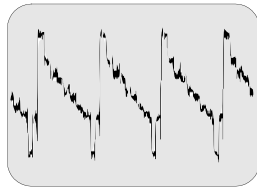
32 A-Board A26 Pin 21 - 1.28V p-p COMB-Y
