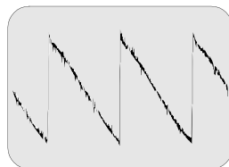
②② A-Bboard A26 Pin 3 - 1.86V p-p NECK PRO
