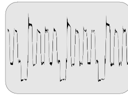
34 A-Board A26 Pin 29 - 5.20V p-p BLUE
