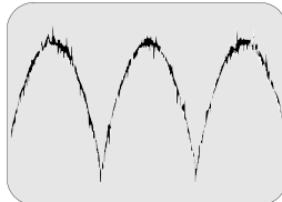
⑬ A-Board A7 Pin 5 - 0.85V p-p V-DAF
