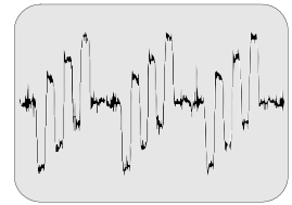
35 A-Board A26 Pin 30 - 0.74V p-p Pb
