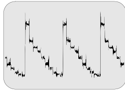
37 A-Board A26 Pin 32 - 0.82V p-p Y
