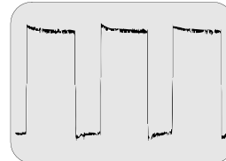
⑭ A-Board A7 Pin 7 - 3.64V p-p H-DAF
