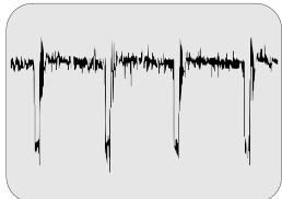
⑥ A-Board A9 Pin 25 - 0.43V p-p TV2 V
