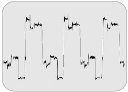
36 A-Board A26 Pin 31 - 4.92V p-p GREEN
