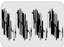
②① A-Bboard A25 Pin 24 - 2.08V p-p SUB V/Y
