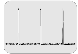
40 A-Board A26 Pin 35 - 3.60V p-p CLP
