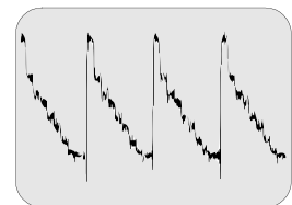
②⑤ A-Bboard A26 Pin 11 - 1.58V p-p SUB V/Y
