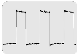
⑦ A-Board A6 Pin 2 - 3.52V p-p H-DRIVE
