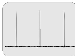
②③ A-Bboard A26 Pin 9 - 4.72V p-p NTSC-VD2
