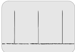
① A-Board IC001 Pin 55 - 3.28V p-p V-SYNC
